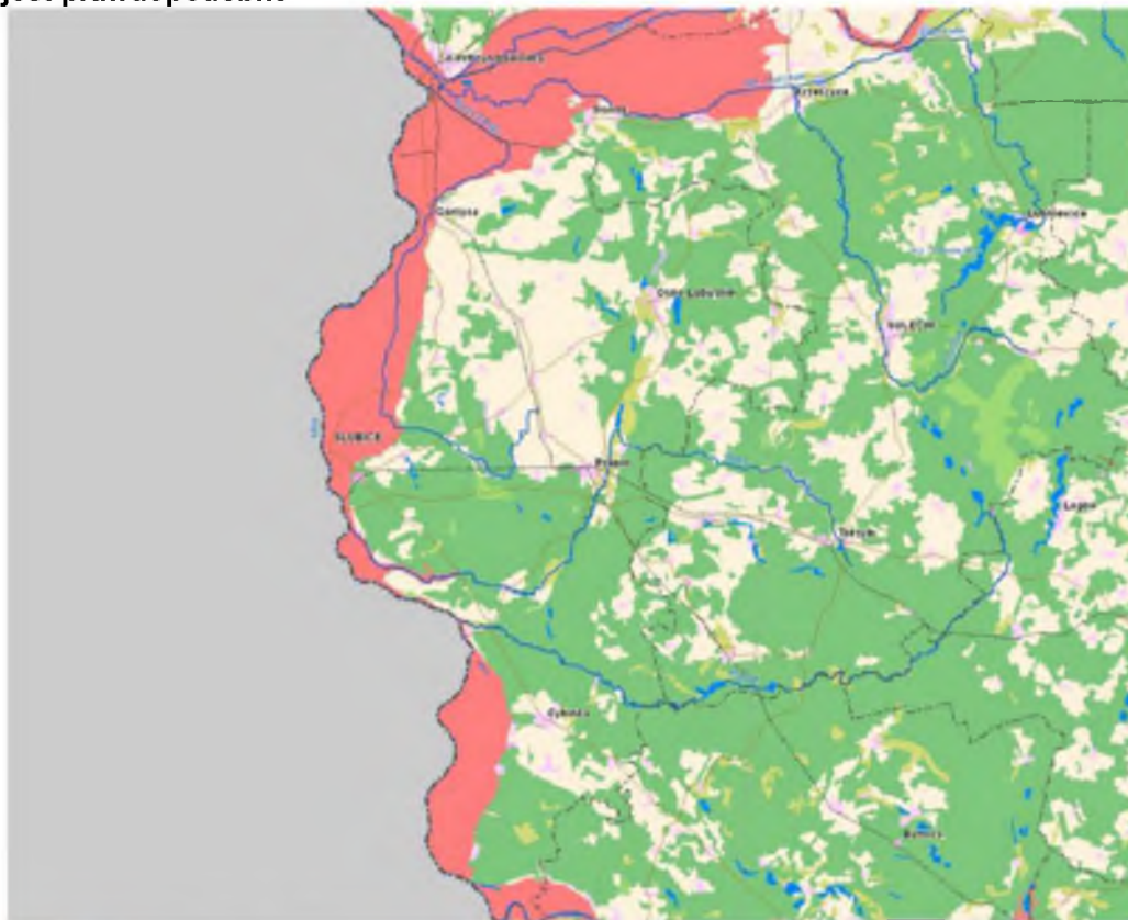
Rysunek 12 Wstępna ocena ryzyka powodziowego – obszary, na których wystąpienie powodzi jest prawdopodobne
