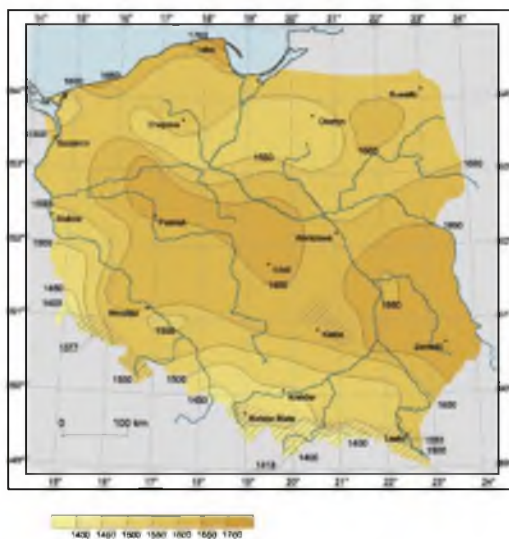
Rysunek 9 Średnie roczne uśłonecznienie w Polsce (w godzinach)
