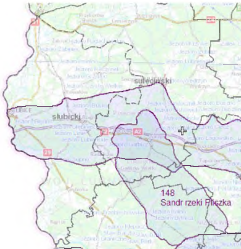
Rysunek 10 Położenie powiatu słubickiego względem głównych zbiorników wód podziemnych GZWP
